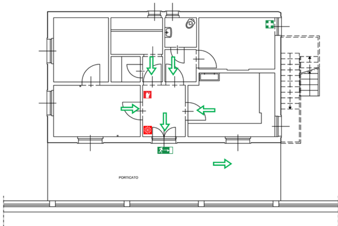
Edificio via Fleming 31/A – piano terra (Microscopia Elettronica)
