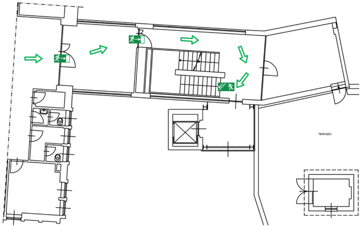
Edificio C 9 – sesto piano
