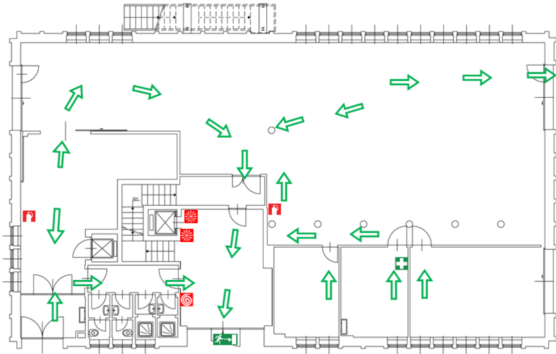
Edificio C 8 – piano terra
