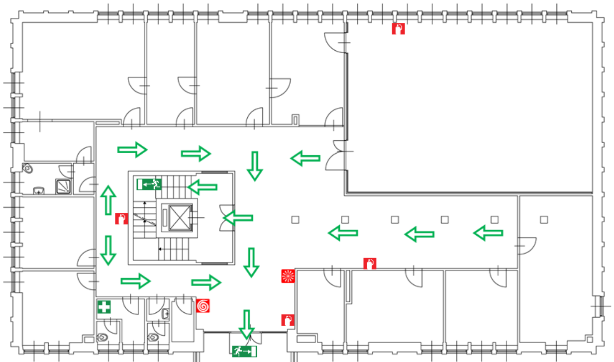
Edificio C 8 – secondo piano
