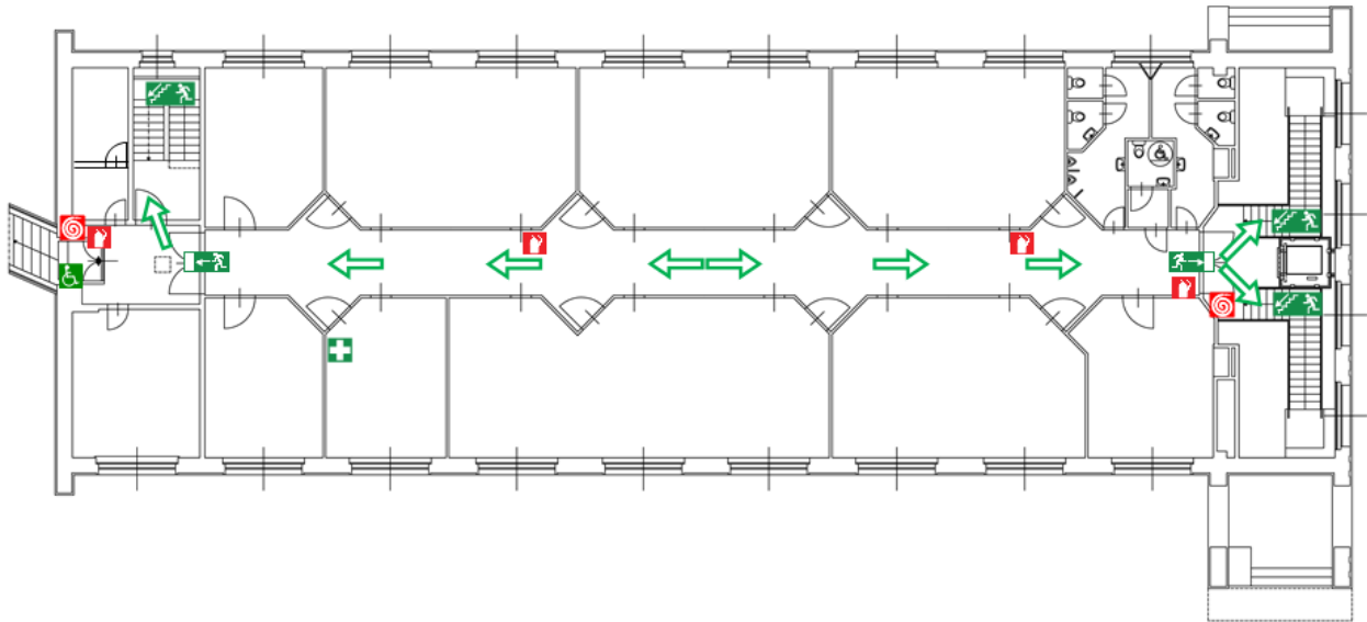
Edificio C 6 – piano soppalco
